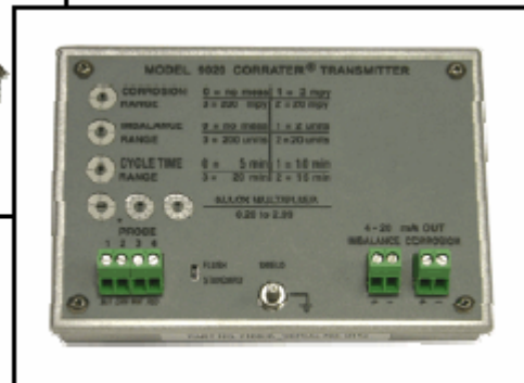
Corrater变送器模块
