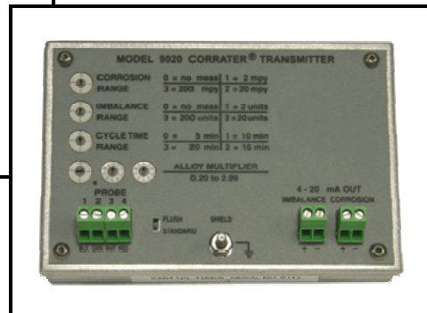
Corratr Transmitter Module
